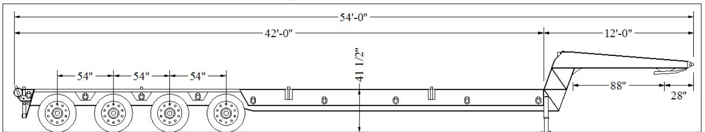
4 AXLE 60 TON SHOWN
