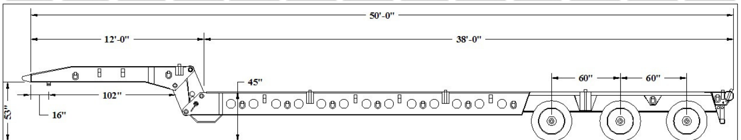
3 AXLE 50 TON SHOWN
