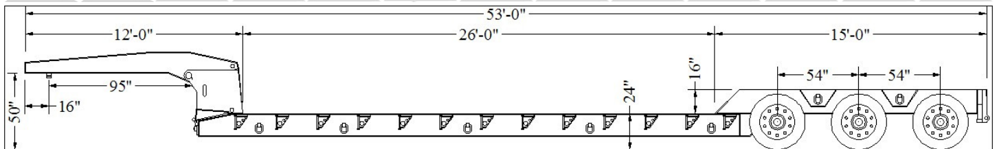
3 AXLE 51 TON SHOWN
